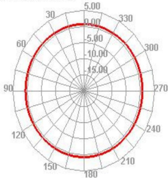
915.000MHz H
