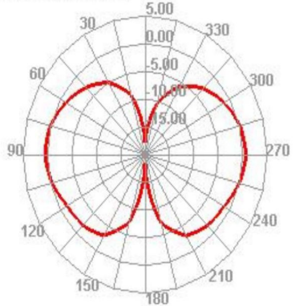
915.000MHz E2
