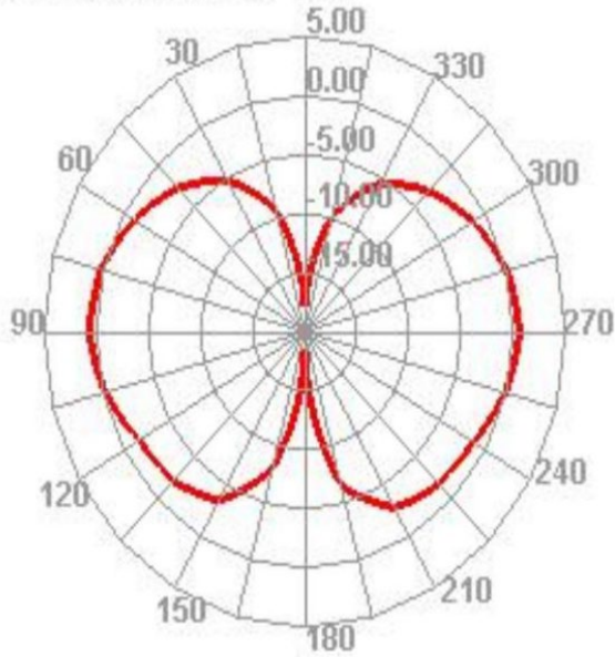
915.000MHz E1
